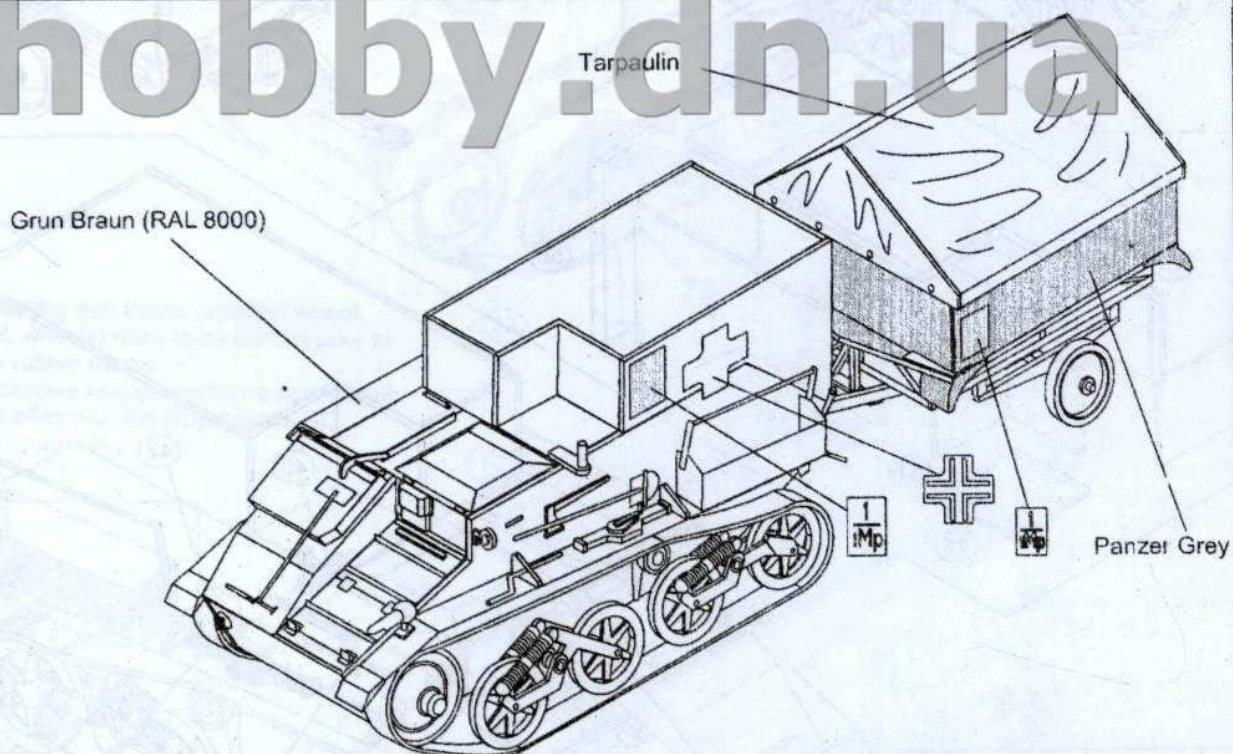
Munitionspanzer auf Fahrgestell Panzerkampfwagen Mk.VI 736(e) - 15 Battery of Art. Battalion, 227 Infantry Division, Belgium or France, late 1941. Подвозчик боеприпасов на шасси танка Mk.VI 736(e) - 15 Батарея 227 Артполка, Бельгия. 1941.
