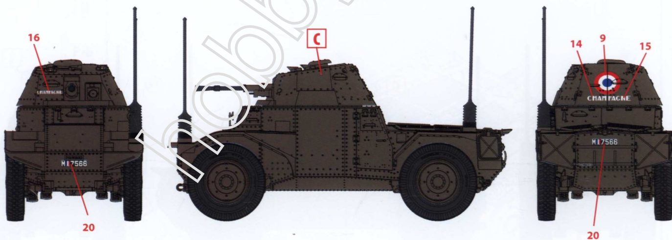
4. Panhard 178 AMD-35, Франция, весна 1940 г. Panhard 178 AMD-35, France, Spring 1940
