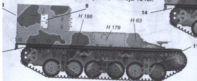
8. Lorraine 38L VBCP, tablice rejestracyjne 11 - 12 z przodu i tyłu pojazdu, Francja 1940r.
