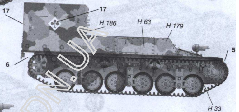
2. Lorraine 38L VBCP, tablice rejestracyjne 5 - 6 z przodu i tyłu pojazdu Francja 1940r.
