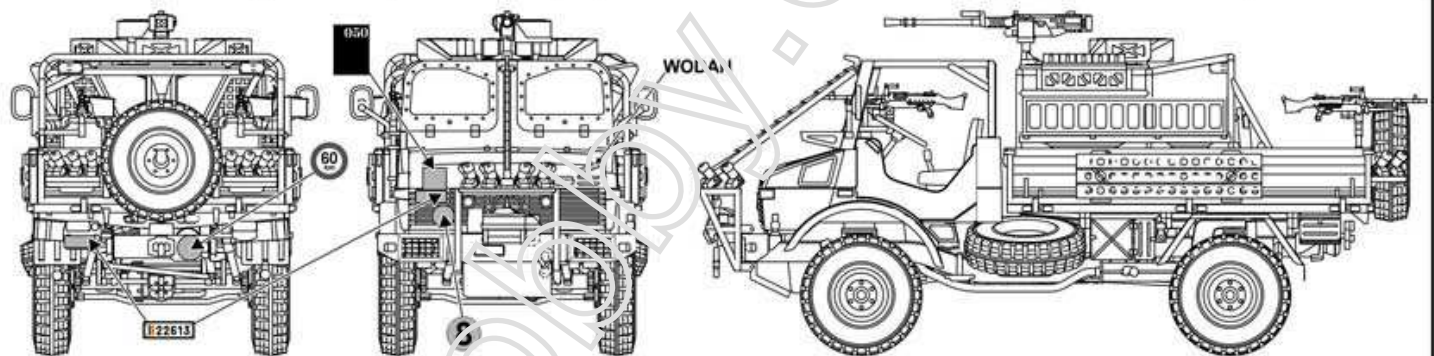
JACAM 4x4 Unimog for long-range patrol missions. Belgian Special Forces. 2016. Olive Green (Close to FS14151) JACAM 4x4 Unimog сил специальных операций Бельгии. 2016. Оливковый. (близко к FS 14151)
