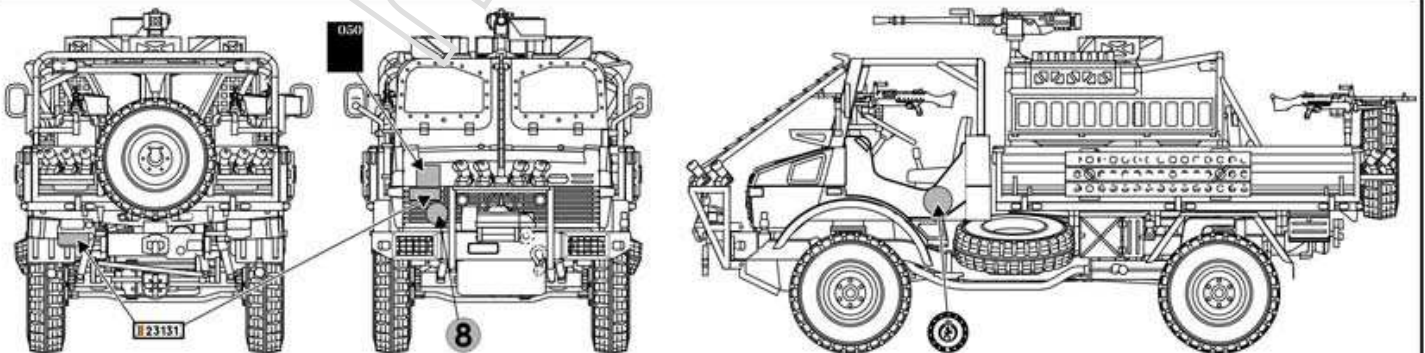
JACAM 4x4 Unimog for long-range patrol missions. Belgian Special Forces. 2018. Olive Green (Close to FS14151) JACAM 4x4 Unimog сил специальных операций Бельгии. 2018. Оливковый. (близко к FS 14151)
