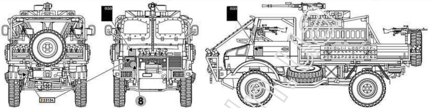
JACAM 4x4 Unimog for long-range patrol missions. Belgian Special Forces. 2016. Sand (Close to FS 23594) JACAM 4x4 Unimog сил специальных операций Бельгии. 2016. Песочный (близко к FS 23594)
