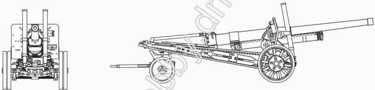
122mm A-19 heavy gun. Red Army 1942. White wash over 4BO (khaki-green). Transport position. 122мм гармата А-19 Червоної Армії, 1942. Білий поверх 4БО. Транспортне положення.
