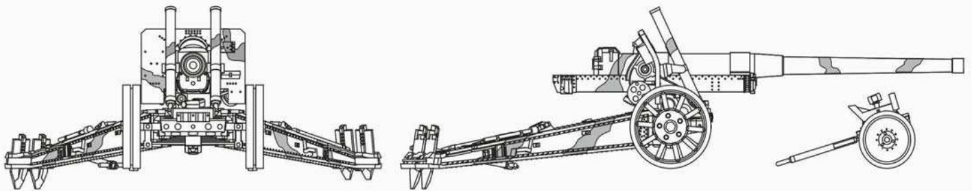
122mm A-19 heavy gun. Red Army 1941. Overall 4BO (khaki-green). Fire position. 122мм гармата А-19 Червоної Армії, 1941. 4БО. Бойове положення.
