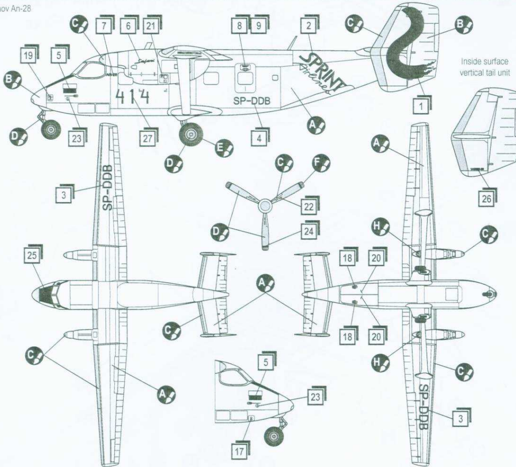
Antonov An-28
