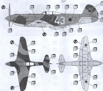
Yak-9U of 153 FAR Air Force USSR, 1944-45 Як-9У 153 ИАП ВВС СССР, 1944-45 г.
