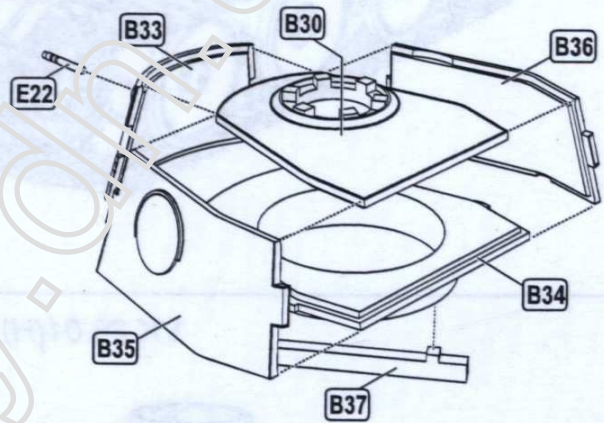
VK 36.01(H) Ausf.H2 turret
