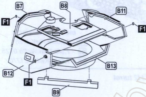
VK 36.01(H) turret
