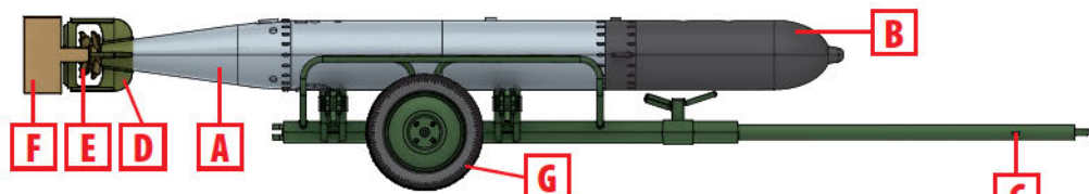
1. Немецкая торпедная тележка с торпедой F5, Вторая мировая война. German Torpedo Trailer with F5 torpedo, World War II
