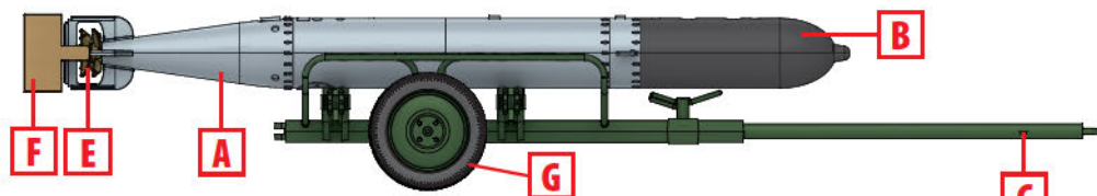
2. Немецкая торпедная тележка с торпедой F5, KG26, Сардиния, 1943 год German Torpedo Trailer with F5 torpedo, KG26, Sardinia, 1943
