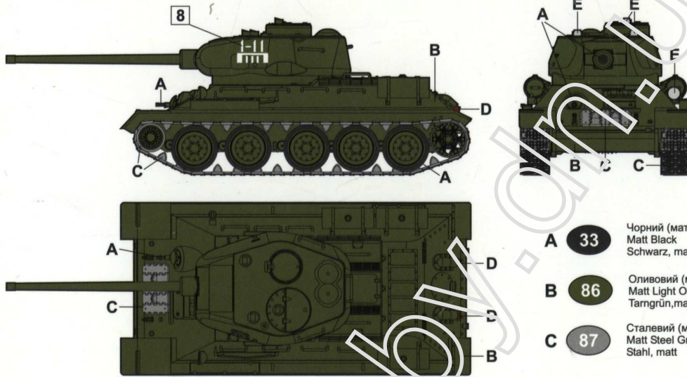
Танк Т-34/85 з гарматою С-53 Tank T-34/85 with S-53 gun
