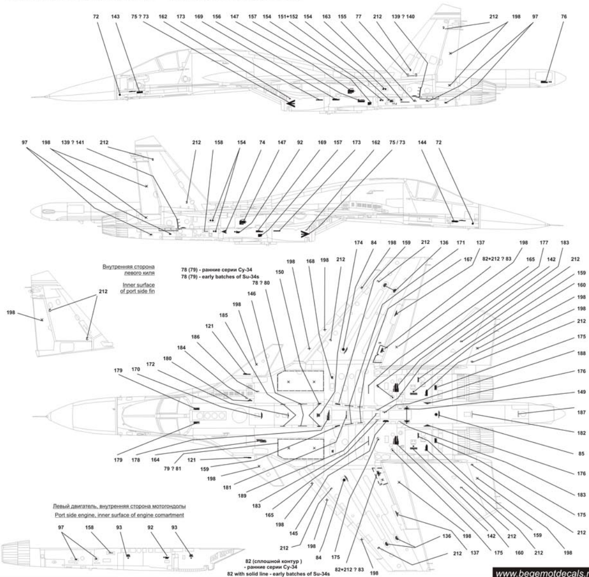
Расположение технических надписей на серийном Су-34 Position of stencil elements on serial Su-34s surfaces.
