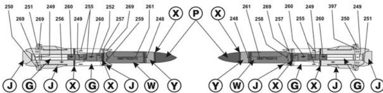
Управляемая ракета "Воздух-Поверхность" X-31П x 6 Kh-31P Air to Surface guided missile x 6
