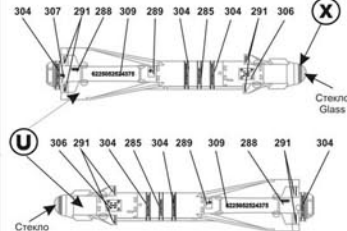
Управляемая ракета "Воздух-Поверхность" типа X-29П x 4 Kh-29P Air to Surface guided missile x 4
