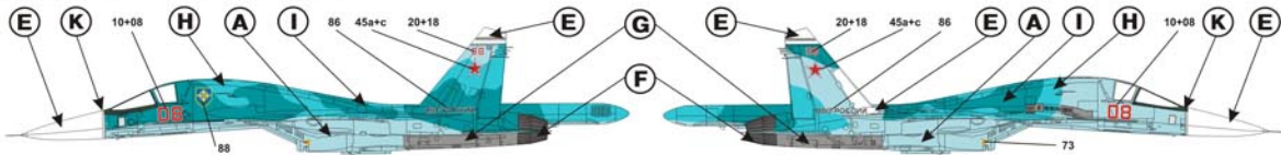
Расположение технических надписей на серийном Су-34 Position of stencil elements on serial Su-34s surfaces.
