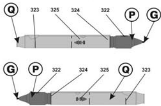
Бомба БETA5-500ШП x 6 BETA5-500ShP bomb x 6
