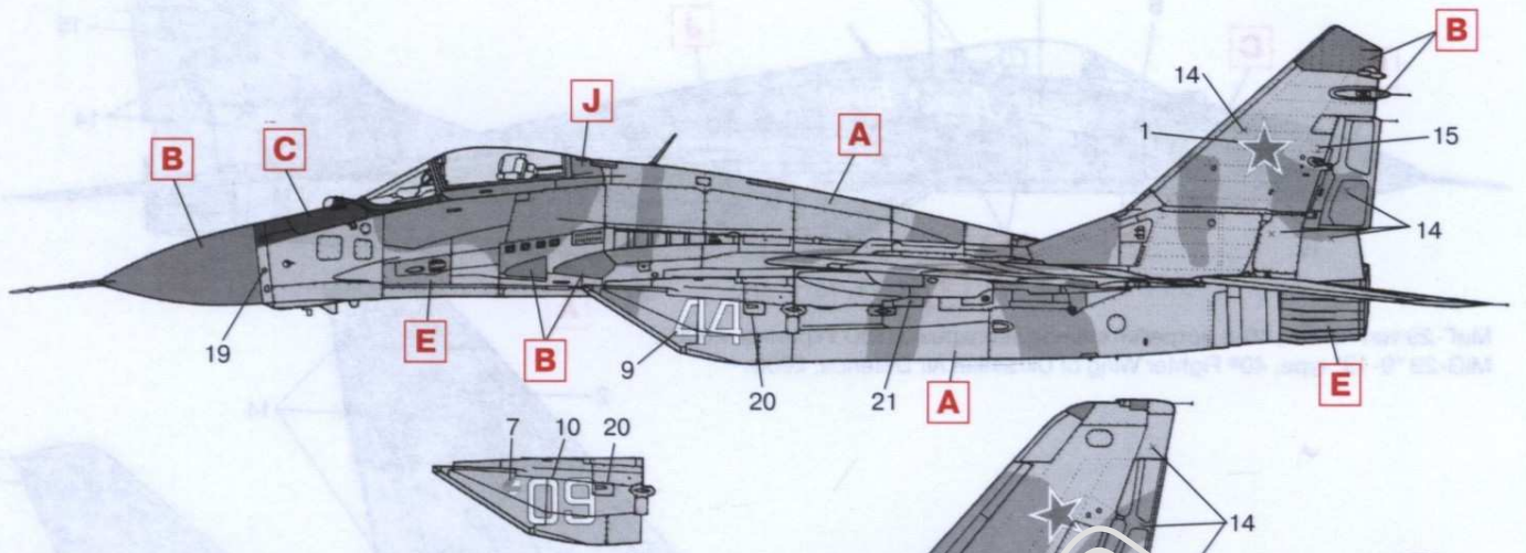
МиГ-29 тип "9-13", 733-й ИАП ВВС России, Дамгартен (Германия), 1994 г. MiG-29 "9-13" type, 733 IAP (Fighter Regiment) of Russian Air Force, Damgarten (Germany), 1994.
