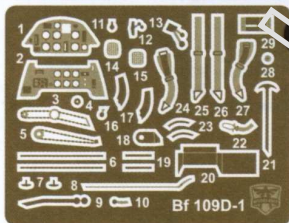
ФОТОЕТЧ ДЛЯ ЗБИРАННЯ МОДЕЛІ PHOTO-ETCHED SHEET FOR ASSEMBLY OF MODEL
