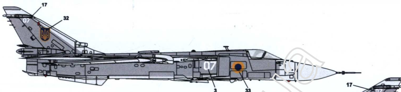
1) Su-24M ВПС України, авіабаза Полтава, літо 1993р. Ukrainian Air Force, Poltava Air Base, summer 1993.
