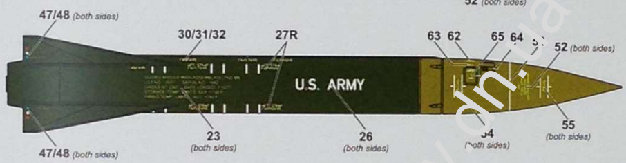
MGM-52 "Lance", армія США MGM-52 "Lance", U.S. Army
