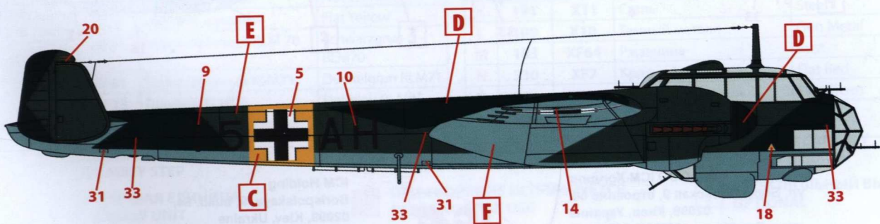
2. Dornier Do 215B-4, 1./Aufkl. Gr.Ob.d.L., Луонетярви, Финляндия, июль 1941 г. Dornier Do 215B-4, 1./Aufkl. Gr.Ob.d.L., Luonetjärvi, Finland, July 1941
