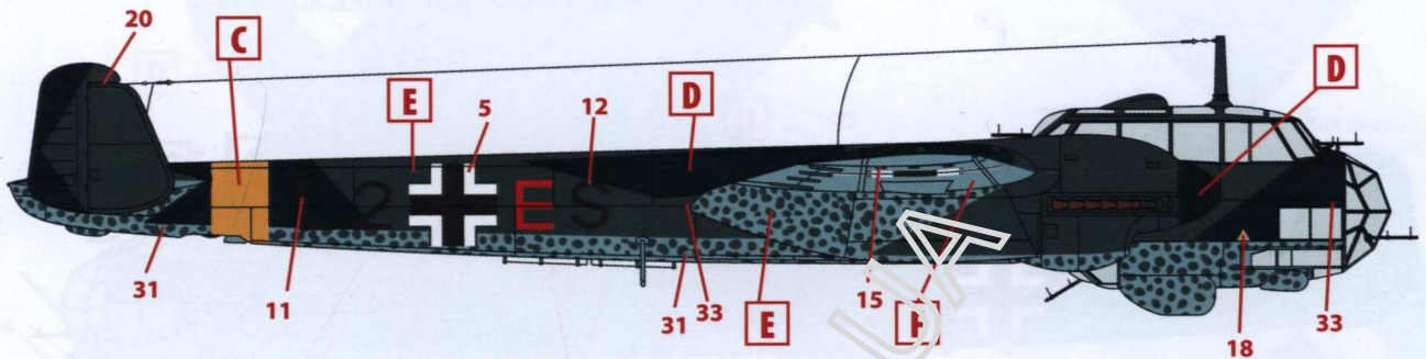
3. Dornier Do 215B-4, 3./Aufkl. Gr.Ob.d.L., Украина, август 1941 г. Dornier Do 215B-4, 3./Aufkl. Gr.Ob.d.L., Ukraine, August 1941
