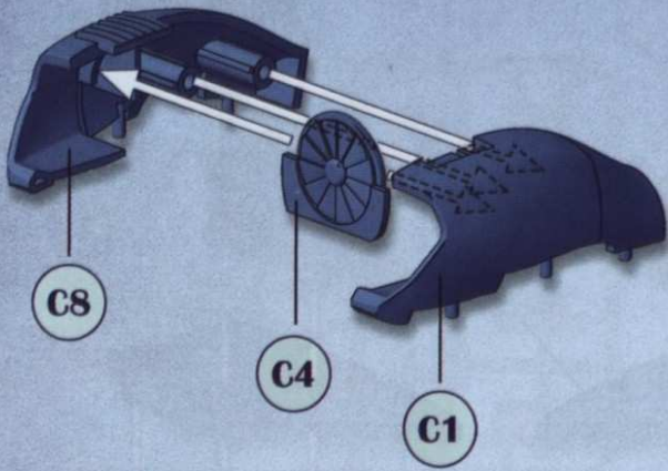
左侧发动机进气道 Left engine air intake
