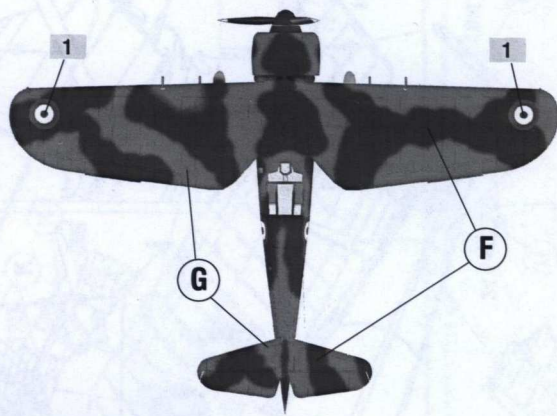
PZL P24F Δ106 z 22 Mira Dioxie (Eskadra myśliwska) lotnisko Wielka Mikra pod Salonikami, wrzesień 1940 roku. w trakcie działań bojowych zdemontowano ostony kół. Patrz: „ZALECANA LEKTURA” nr 1, 2, 3 i 5. PZL P24F Δ106, 22 Mira Dioxie (Fighter Squadron), Great Micra Airfield Thessalonika, September 1940. Wheel fairings removed during service. See: “Suggested reading” No 1, 2, 3 and 5.
