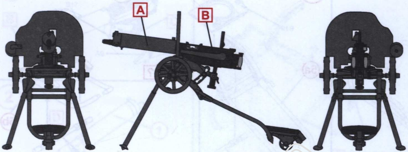
Пулемет «Максим» обр. 1910 г. в положении для стрельбы сидя. Maxim machine gun (1910) in firing seating position.
